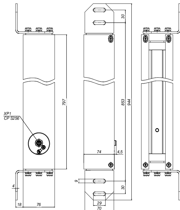
Габаритный чертеж Стойка излучателей (приемников)
